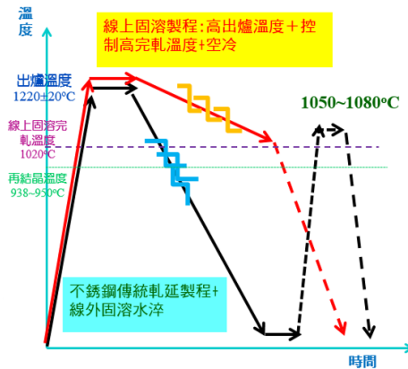
不銹鋼線上固溶與線外固溶製程之示意圖(詳見內文第一篇)
